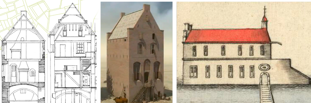
Fig. 8 Steenhuis en Borg; v.l.n.r.: dwarsdoorsnede van het steenhuis te Bunderhee (7.60 x 11.40; hoogte 15,4 meter); dwarsdoorsnede van het uitstekend bewaarde steenhuis, eerste bouwphase van het Hinckaertshuis in stad Groningen (ca. 1300; 7.8 x 14.8; hoogte 17.5 meter, met dank aan Taco Tel; Tel 2012); een gereconstrueerd aanzicht van het Hinckaertshuis rond 1300 en aanzicht van Borg Harssens II, van oorsprong rond 1550.
